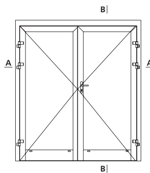
Rys. 10. Drzwi dwuskrzydłowe aluminiowe bez przegrody termicznej, z progim.
