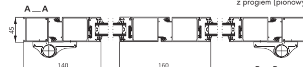
Rys. 12. Przekrój drzwi dwuskrzydłowych aluminiowych bez przegrody termicznej (poziomy).
