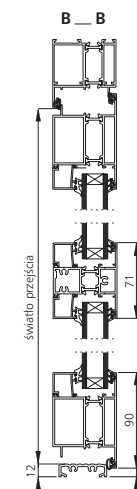
Rys. 14. Przekrój drzwi aluminiowych z przegrodą termiczną (pionowy).
