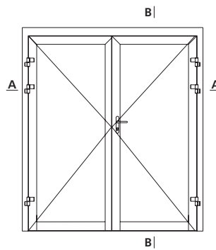
Rys. 13. Drzwi dwuskrzydłowe aluminiowe z przegrodą termiczną, z progim.
