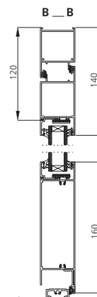
Rys. 11. Przekrój drzwi dwuskrzydłowych aluminiowych bez przegrody termicznej, z progim (pionowy).
