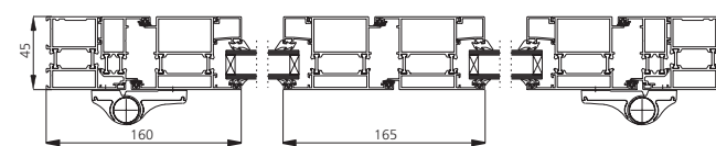
Rys. 15. Przekrój drzwi dwuskrzydłowych aluminiowych z przegrodą termiczną (poziomy).
