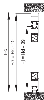
Rys. 106. Montaż w otworze - przekrój pionowy - drzwi jednoskrzydłowe - system AW45.
