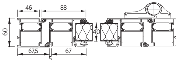
Rys. 7. Przekrój poziomy przez drzwi aluminiowe z przegrodą termiczną DoorPro 60 (drzwi wypełnione panelem stalowym 40 [mm]) - system MB 60E.
