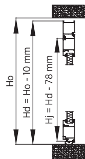
Rys. 111. Montaż w otworze – przekrój pionowy – drzwi jednoskrzydłowe – system MB45.
