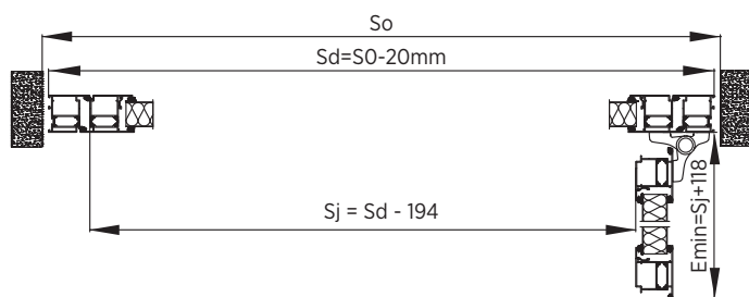
Rys. 101. Montaż w otworze - przekrój poziomy - drzwi jednoskrzydłowe - system MB60E.
