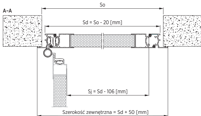
Rys. 112. Zależności wymiarowe – przekrój poziomy – drzwi jednoskrzydłowe – system AW45 z ościeżnicą narożną.
