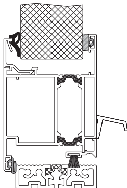
Rys. 91. Drzwi DoorPro 60 otwierane do wewnątrz.
