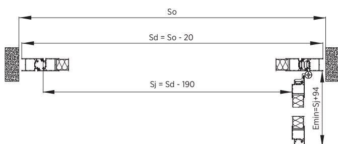
Rys. 104. Montaż w otworze - przekrój poziomy - drzwi jednoskrzydłowe - system AW45.
