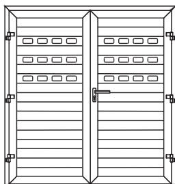
Rys. 77. Drzwi aluminiowe dwuskrzydłowe wypełnione profilem aluminiowym AW 100, przeszklewane.
