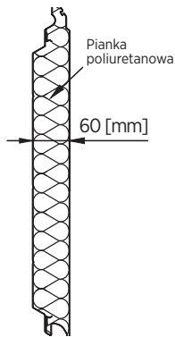
Rys. 15. Panel stalowy 60 [mm] bez przetłoczeń (G).
