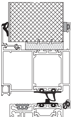
Rys. 83. Drzwi DoorTherm 86 otwierane na zewnątrz.
