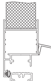
Rys. 93. Drzwi DoorPro 45 otwierane do wewnątrz.
