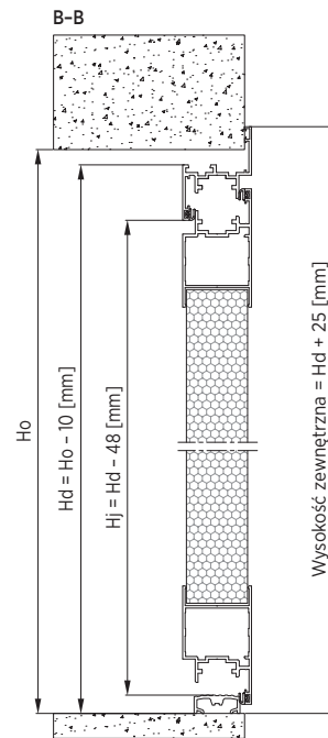
Rys. 113. Zależności wymiarowe – przekrój pionowy – drzwi jednoskrzydłowe – system AW45 z ościeżnicą narożną.
