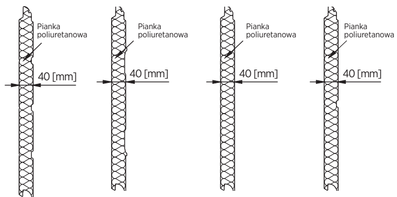
Rys. 19. Panel stalowy 40 [mm] przetłoczeniami niskimi (N).
