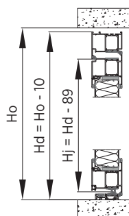
Rys. 89. Montaż w otworze - przekrój pionowy - drzwi jednoskrzydłowe - system MB86N ST.
