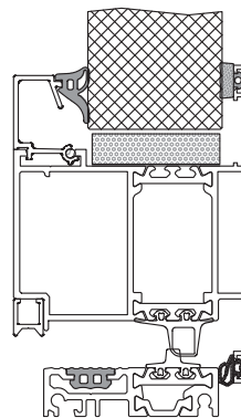
Rys. 85. Drzwi DoorPro 70 otwierane na zewnątrz.
