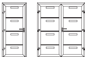
Rys. 70. Aplikacje ozdobne AP-1 w drzwiach jedno- i dwuskrzydłowych.
