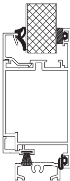
Rys. 94. Drzwi DoorLight 45 otwierane na zewnątrz.
