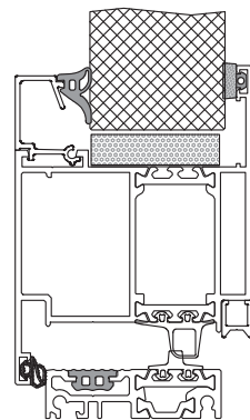
Rys. 86. Drzwi DoorPro 70 otwierane do wewnątrz.
