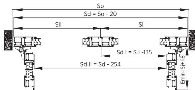
Rys. 102. Montaż w otworze - przekrój poziomy - drzwi dwuskrzydłowe - system MB60E.
