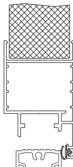
Rys. 92. Drzwi DoorPro 45 otwierane na zewnątrz.
