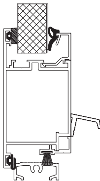
Rys. 95. Drzwi DoorLight 45 otwierane do wewnątrz.
