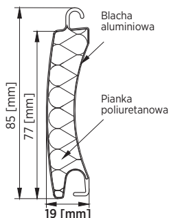
Rys. 27. Profil AW 77.
