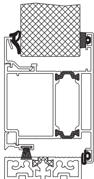
Rys. 90. Drzwi DoorPro 60 otwierane na zewnątrz.
