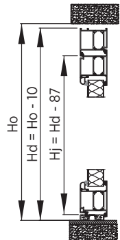
Rys. 100. Montaż w otworze – przekrój pionowy – drzwi jednoskrzydłowe – system MB70 RC.
