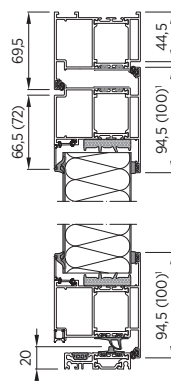
Rys. 2. Przekrój pionowy przez drzwi aluminiowe z przegrodą termiczną DoorTherm 86 (drzwi wypełnione panelem stalowym 60 [mm]) - system MB86N ST.
