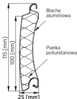
Rys. 29. Profil AW 100.
