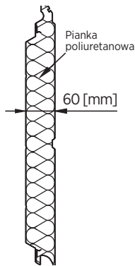
Rys. 16. Panel stalowy 60 [mm] z przetłoczeniami wysokimi (W).
