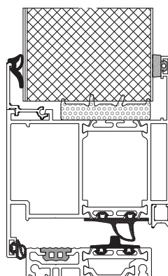
Rys. 84. Drzwi DoorTherm 86 otwierane do wewnątrz.
