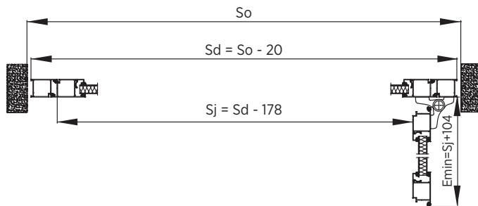
Rys. 109. Montaż w otworze – przekrój poziomy – drzwi jednoskrzydłowe – system MB45.
