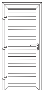
Rys. 26. Drzwi aluminiowe z profilem AW 77.
