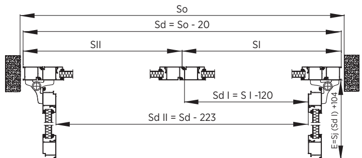
Rys. 110. Montaż w otworze – przekrój poziomy – drzwi dwuskrzydłowe – system MB45.
