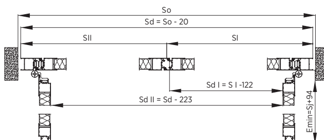
Rys. 105. Montaż w otworze - przekrój poziomy - drzwi dwuskrzydłowe - system AW45.
