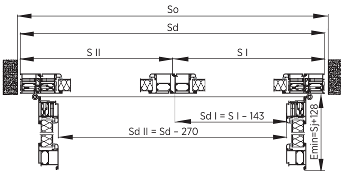
Rys. 99. Montaż w otworze – przekrój poziomy – drzwi dwuskrzydłowe – system MB70 RC.
