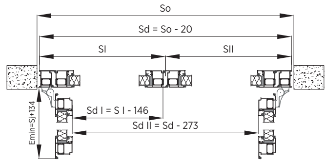
Rys. 97. Montaż w otworze – przekrój poziomy – drzwi dwuskrzydłowe – system MB79N ST.
