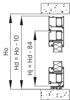
Rys. 98. Montaż w otworze – przekrój pionowy – drzwi jednoskrzydłowe – system MB79N ST.
