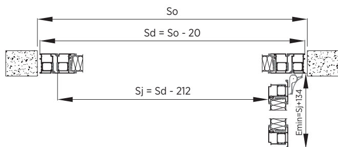
Rys. 87. Montaż w otworze - przekrój poziomy - drzwi jednoskrzydłowe - system MB86N ST.
