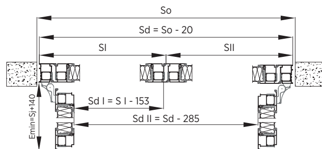
Rys. 88. Montaż w otworze - przekrój poziomy - drzwi dwuskrzydłowe - system MB86N ST.
