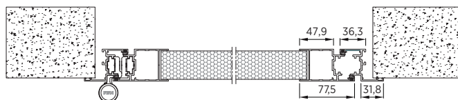
Rys. 11. Przekrój poziomy przez drzwi bez przegrody termicznej DoorPro 45 (drzwi wypełnione panelem stalowym 40 [mm]) - system AW 45 z ościeżnicą narożną
