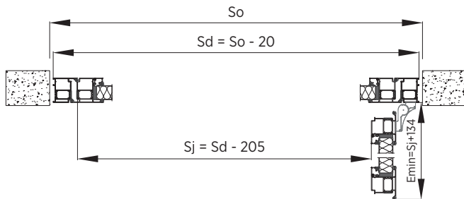
Rys. 96. Montaż w otworze – przekrój poziomy – drzwi jednoskrzydłowe – system MB79N ST.
