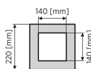
Rys. 67. Typ AP-3, wymiar 220x220 [mm].
