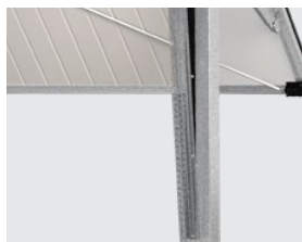
Sistema di molle a trazione responsabile per il bilanciamento del peso dell'anta
