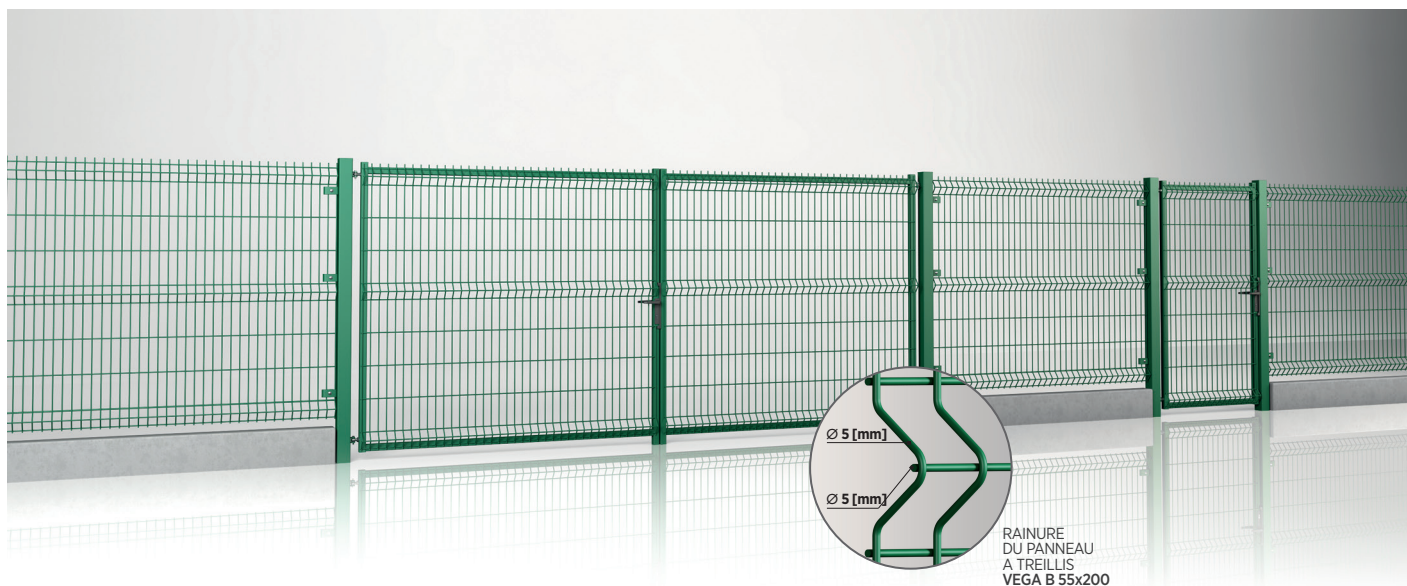
Clôturesystème avec portail et portillon MODEST avec remplissage en panneaux à treillis VEGA B, maille 55x200
