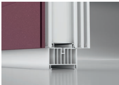
Montážní a přepravní profil
