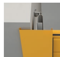
Montáž do stavebního otvoru – maskující prvek před otvorem
