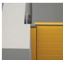
Montáž za stavebním otvorem – maskující prvek za otvorem
