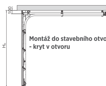
Montáž za stavebním otvorem - kryt za otvorem
