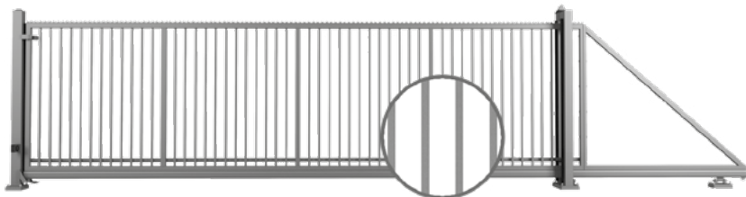
POSUVNÁ BRÁNA S VÝPLNÍ V PODOBĚ UZAVŘENÝCH PROFILŮ 25 X 25 [MM], PŘIVAŘENÝCH KE KONSTRUKCI - POHLED ZE STRANY NEMOVITOSTI.
