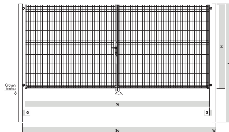
Dvoukřídlová brána MODEST pohled zevnitř
