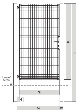
Branka MODEST pohled zevnitř
