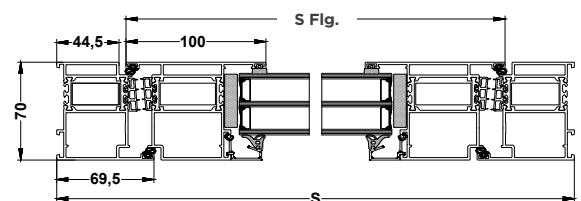
Rahmen K520131, Flügel K520146
