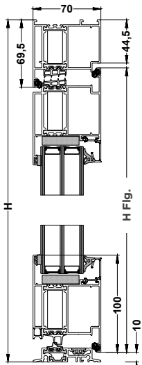
Rahmen K520130, Flügel K520144
