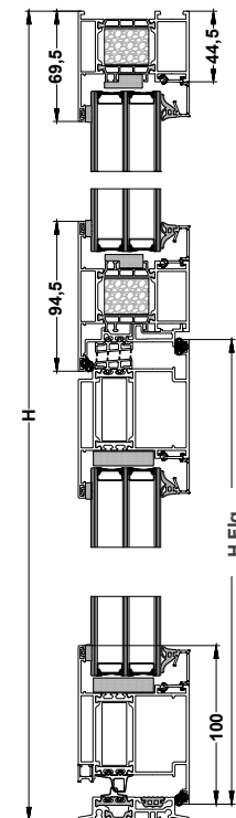
Rahmen K520012, Flügel K520144, Querholm K520052
