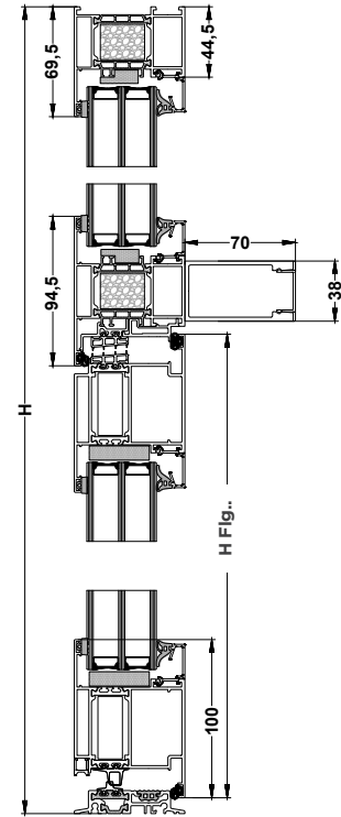
Rahmen K520012, Flügel K520144, Querholm K520052 + Verstärkung K413923 von innen
