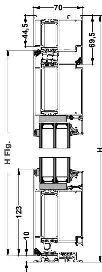
Rahmen K520131, Flügel K520150
