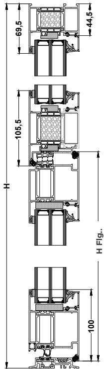
Rahmen K520012, Flügel K520144, Querholm K520053
