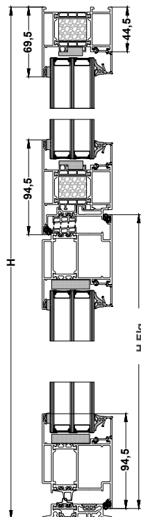
Rahmen K520012, Flügel K520140, Querholm K520052
